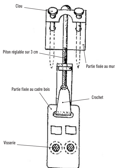
Crochet ajustable pour cadre bois
