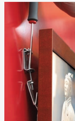
Ajuster le cadre avec la vis de réglage à l'aide d'un tournevis cruxiforme
